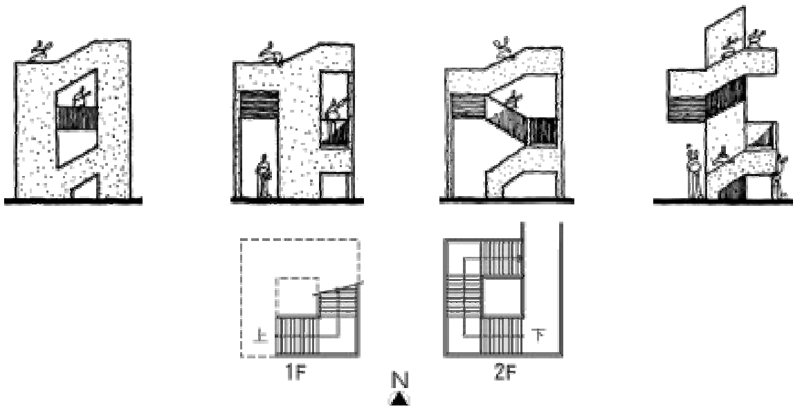
圖(六) 一、二樓樓梯平面圖
